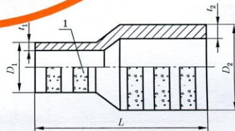
b) 挤压异径型套筒
