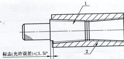
图 5 直螺纹套筒螺纹中径止端检验示意图
