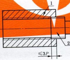
图 4 直螺纹套筒螺纹中径通端检验示意图
